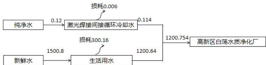
图 2-1 项目水平衡图 t/a
