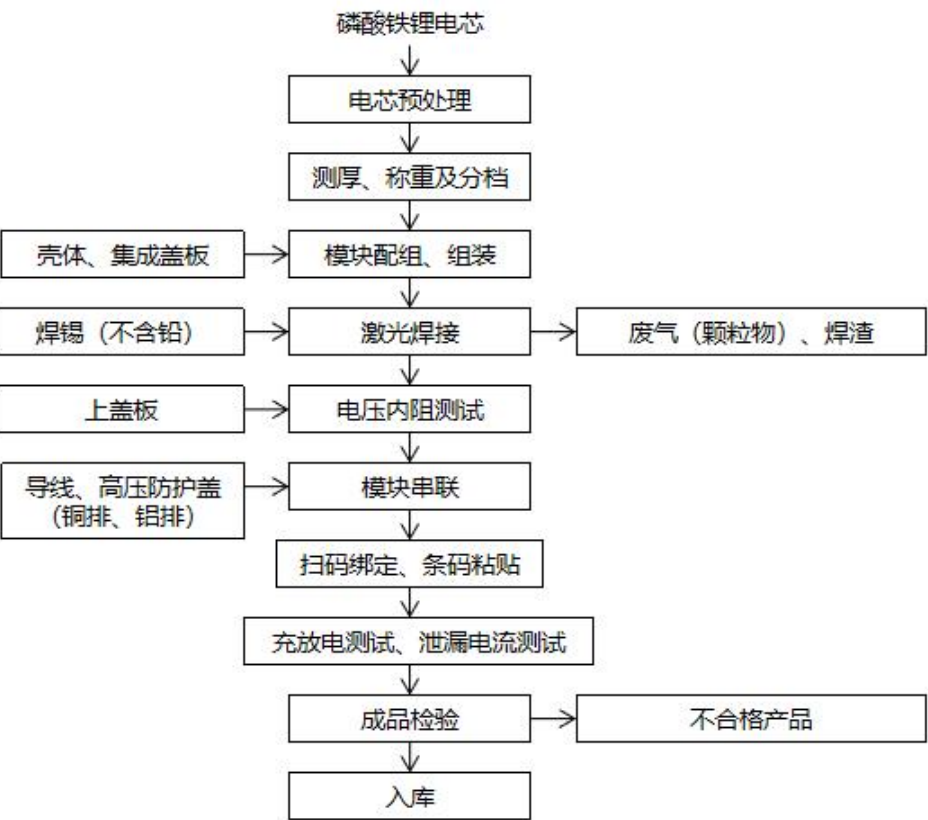
图 2-2 磷酸铁锂电池包装组生产工艺流程及产污节点图
