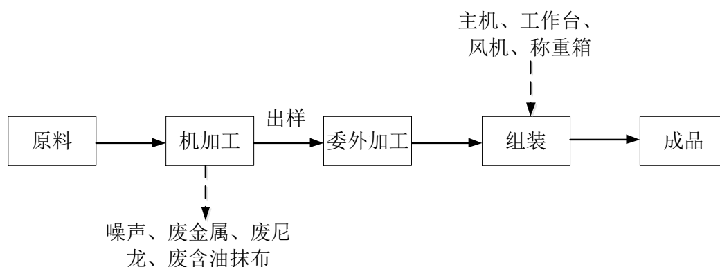
图 5-1 项目生产工艺流程及产污节点图
