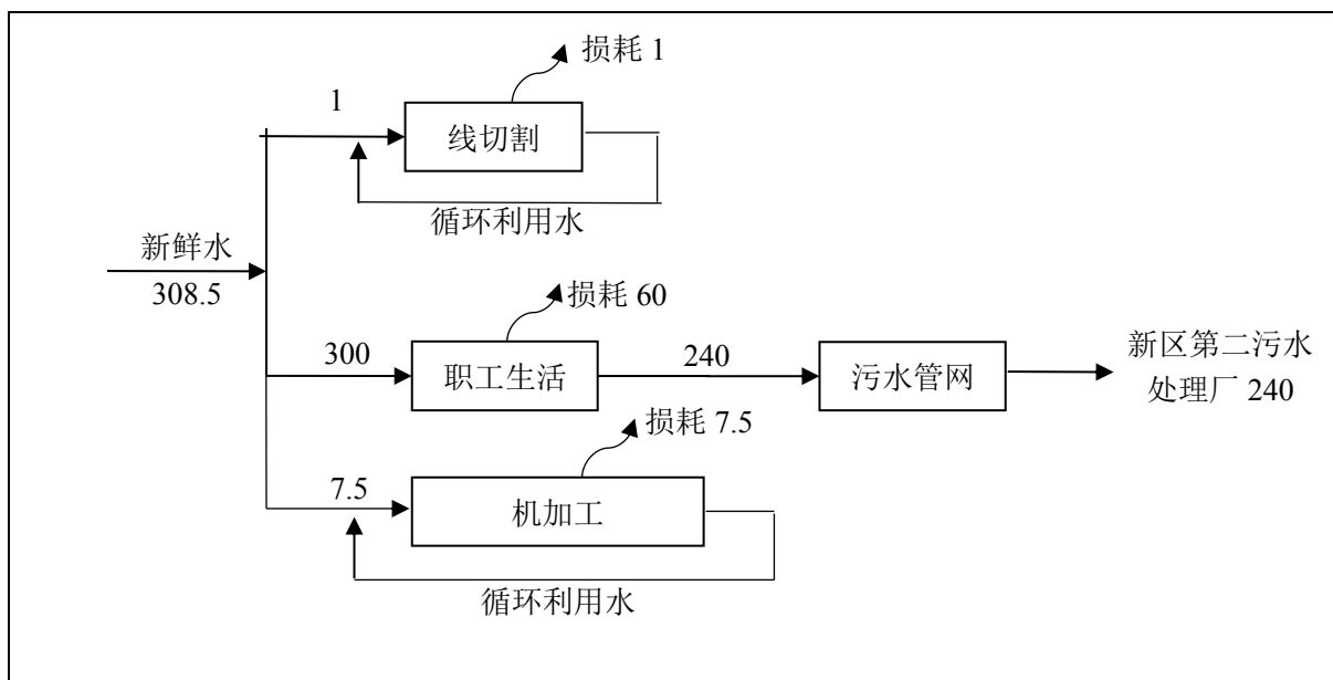
图 5-2 本项目水平衡图 (t/a)
