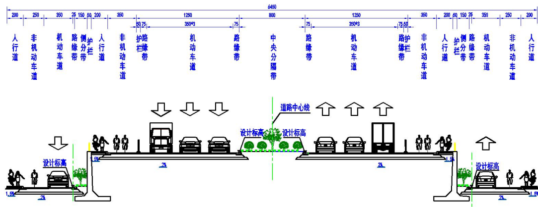
图 1-5 通浒桥两侧辅道横断面图
