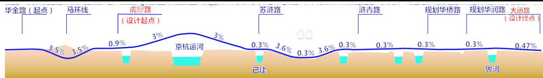
图 1-3 路线纵断面图
