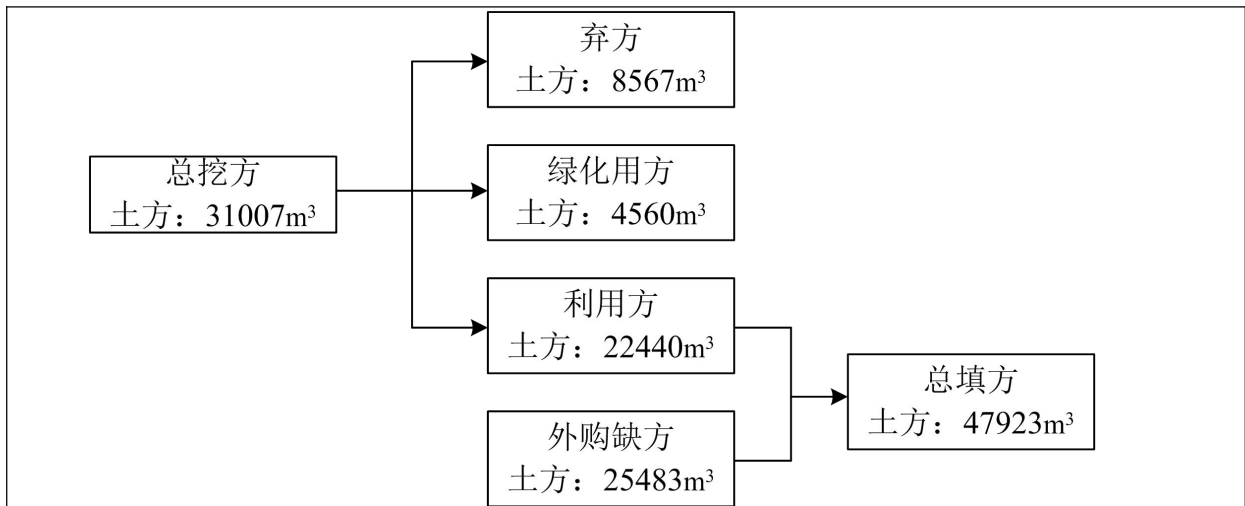
图 1-6 拟建项目路基工程土石方平衡图
