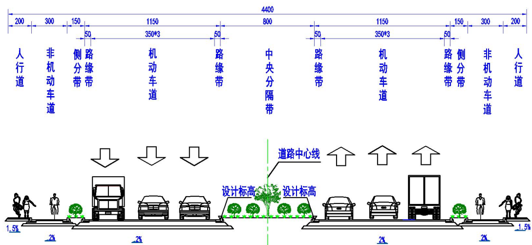
图 1-4 道路标准横断面图
