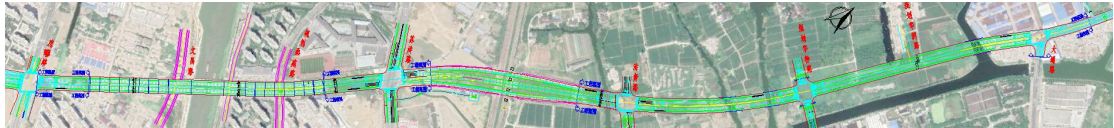
图 1-1 路线平面图
