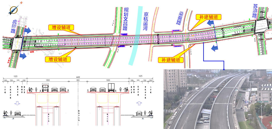
图 1-2 通浒桥两侧辅道平面图
